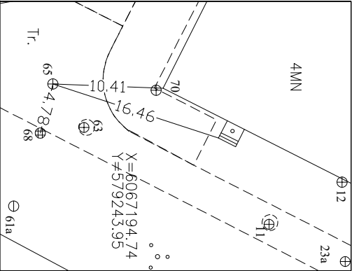
PRIEŠIMO BRĖŽINYS
