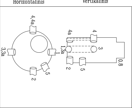
ŠULINIO PLOVIMAI (Matmenys duoti m)
