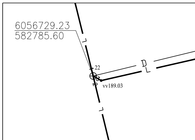
Pririšimo brėžinys
