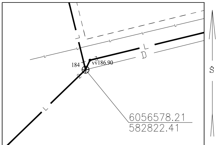
Pririšimo brėžinys
