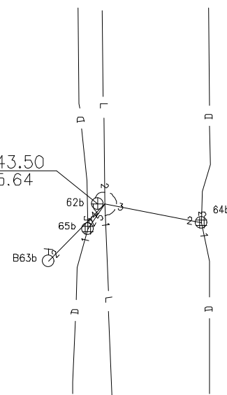
Pririšimo brėžinys
