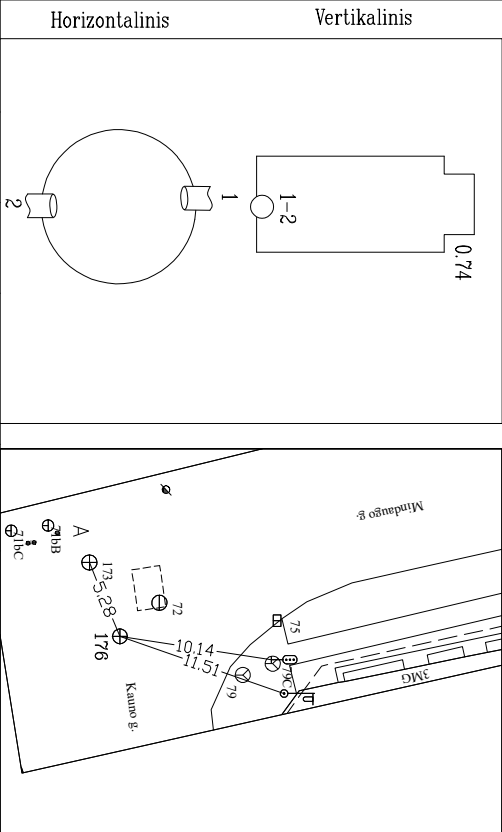
ŠULINIO PLOVIAI (Matmenys duoti m) PRIEŠIMO BRĖŽINYS
