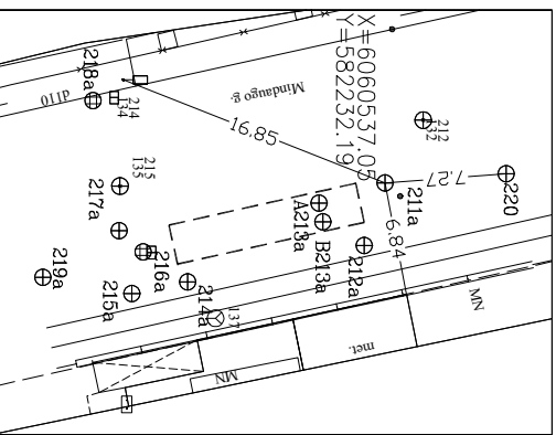
PRIEŠIMO BRĖŽINYS
