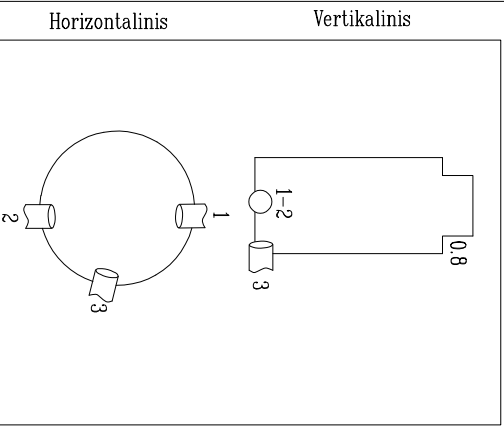
ŠULINIO PĖJIVIAI (Matmenys duoti m)
