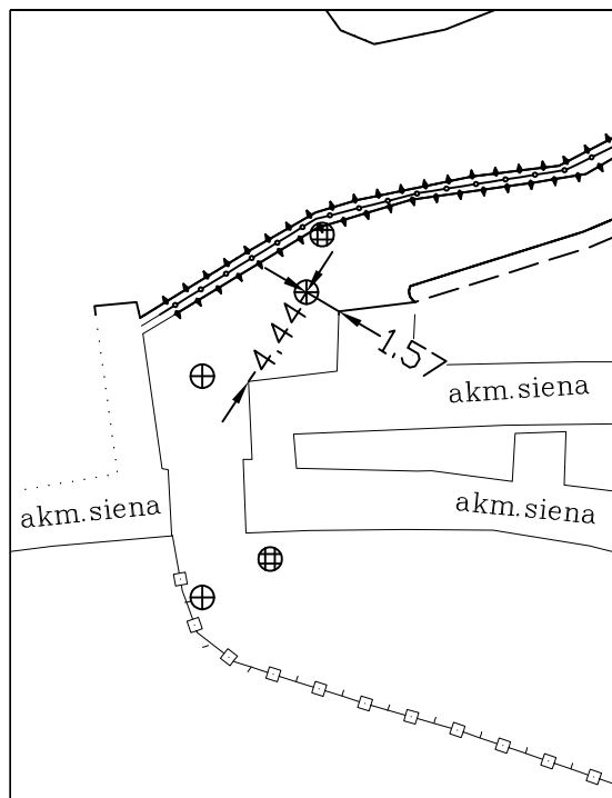
PRIRIŠIMO BRĖŽINYS
