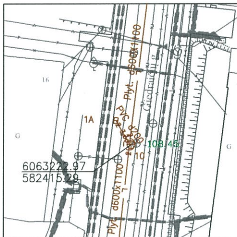
Pririšimo brėžinys
