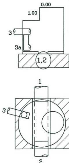
Šulinio pjūviai
