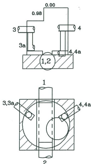
Šulinio pjūviai
