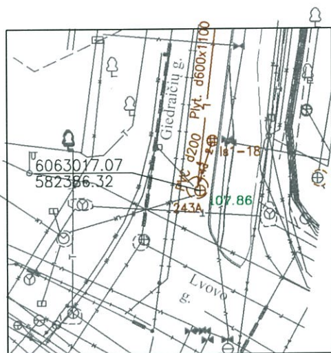
Pririšimo brėžinys
