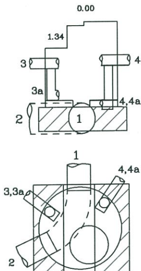
Šulinio pjūviai
