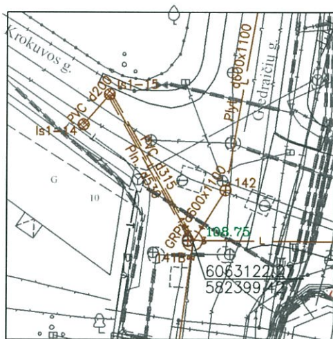
Pririšimo brėžinys
