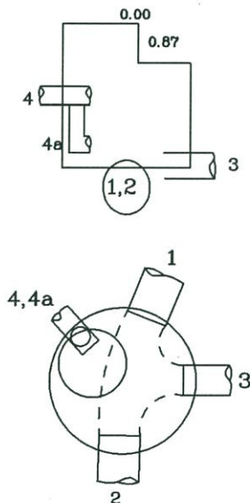
Šulinio pjūviai
