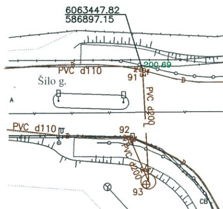
Pririšimo brėžinys
