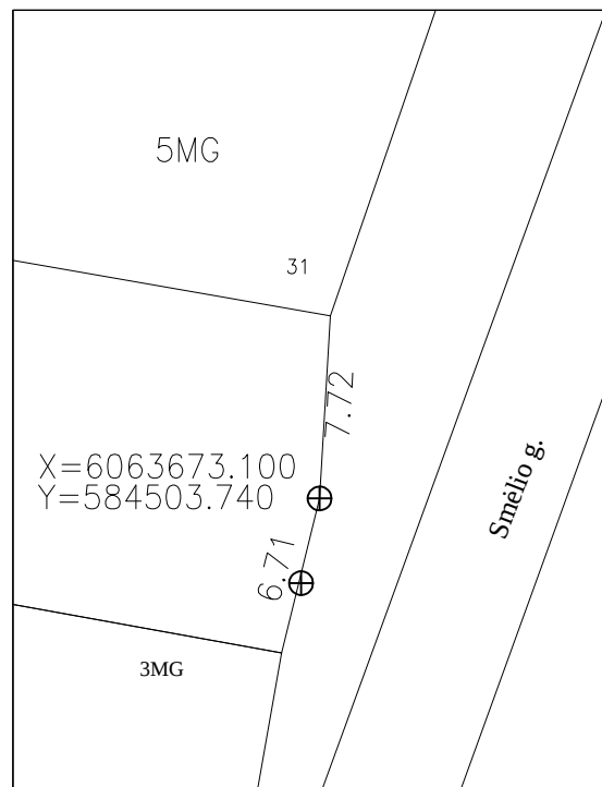
PRIRIŠIMO BRĖŽINYS
