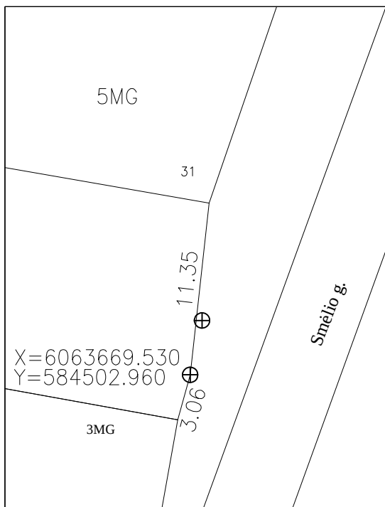
PRIRIŠIMO BRĖŽINYS
