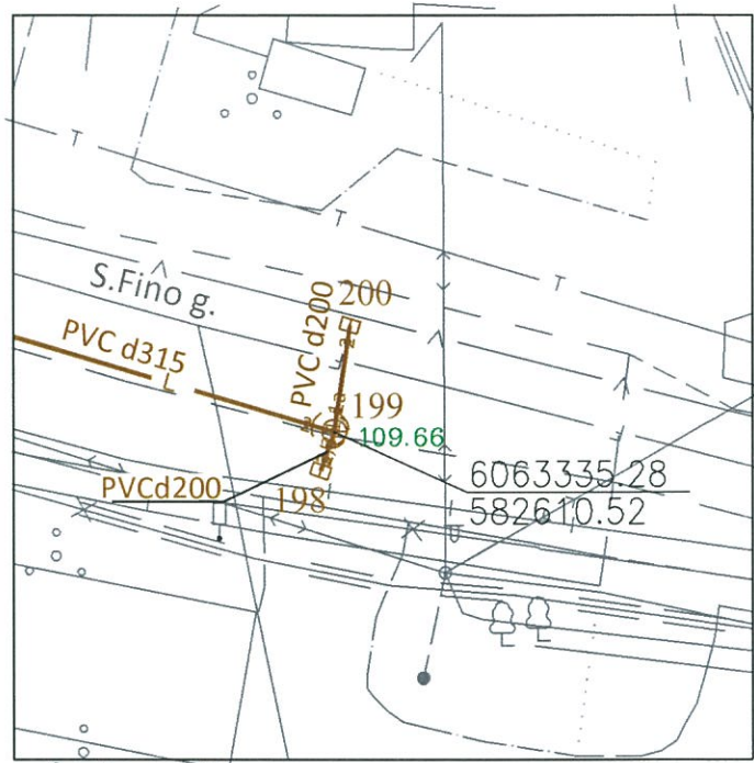
Pririšimo brėžinys
