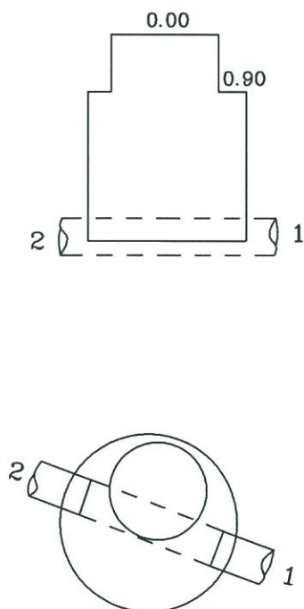
Šulinio pjūviai
