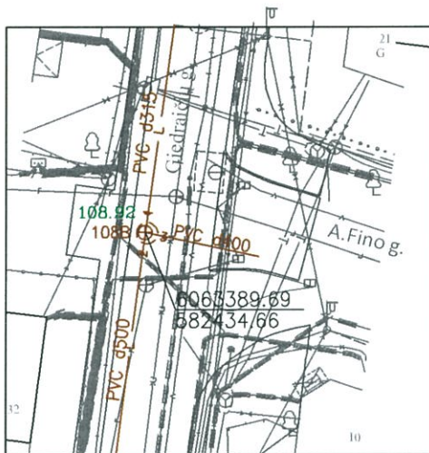
Pririšimo brėžinys
