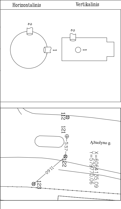
ŠULINIO PĖŲVIAI (Mažmenys duoti m)PRIRIŠIMO BRĖŽINYS
