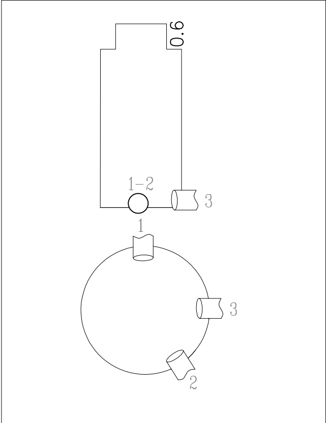
ŠULINIO PJŪVIAI (Matmenys duoti m)
