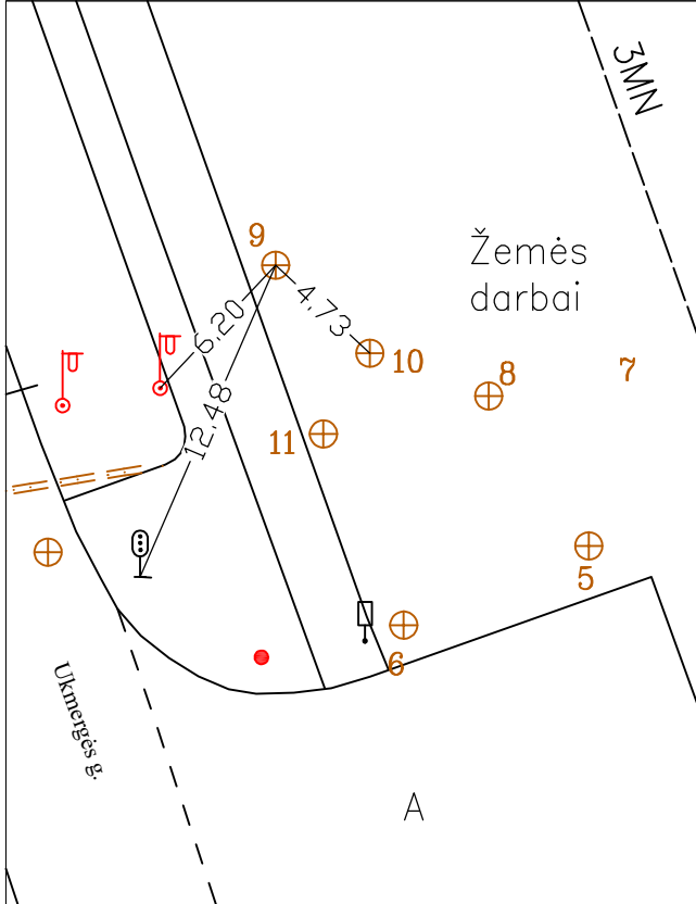
PRIRIŠIMO BRĖŽINYS
