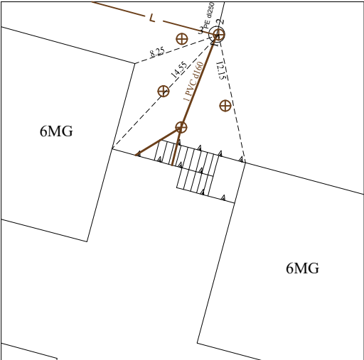
Prižišimo brėžinys
