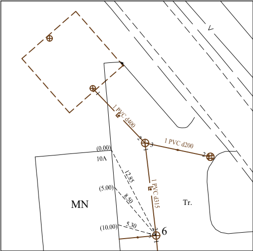
Pririšimo brėžinys
