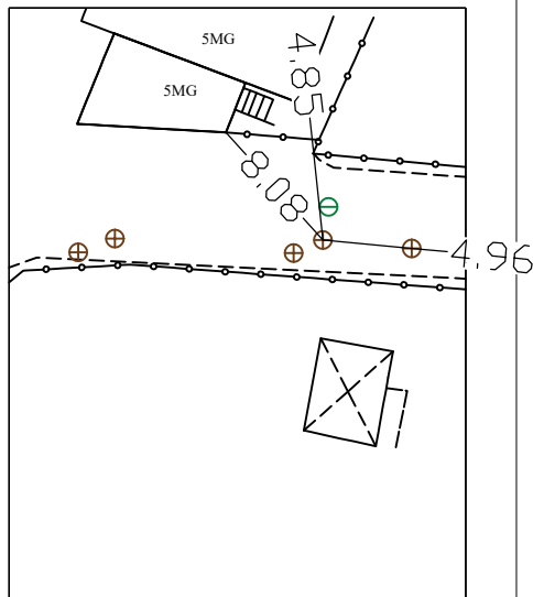
PRIRIŠIMO BRĖŽINYS
