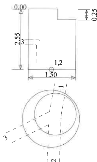
Šulinio pjūviai
