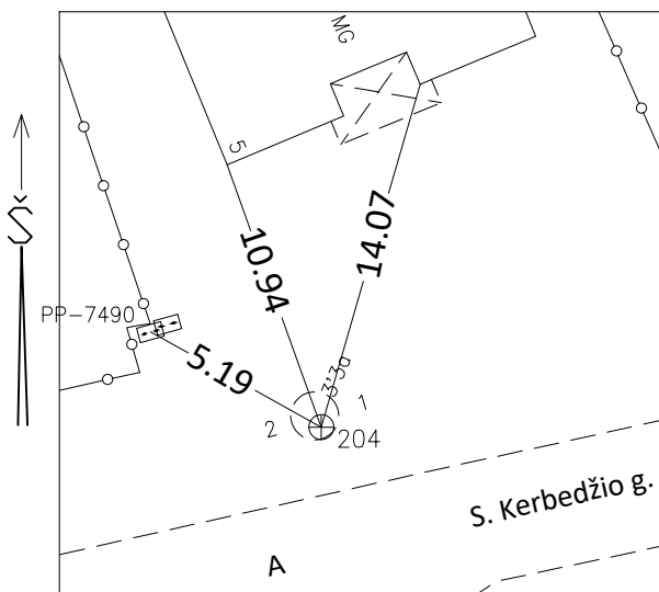
Pririšimo schema
