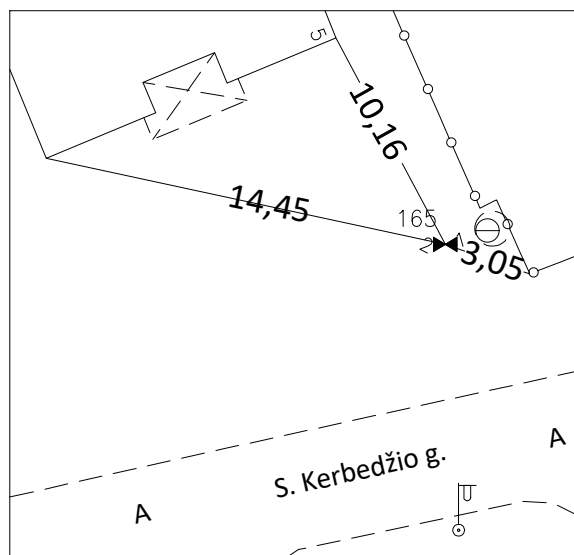
Pririšimo schema
