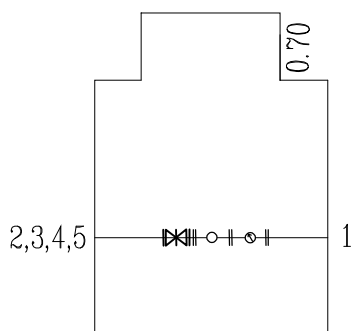
ŠULINIO PJŪVIAI (Matmenys duoti m)
