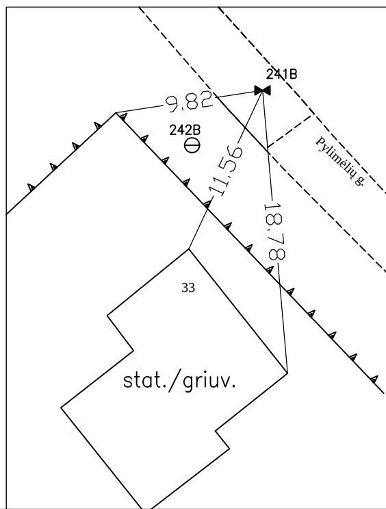
PRIRIŠIMO BRĖŽINYS
