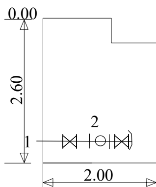
Šulinio pjūviai
