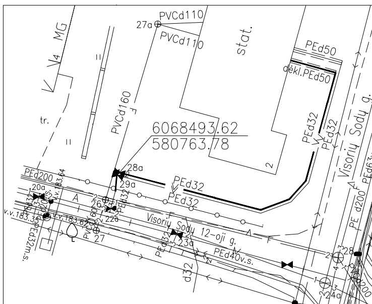
PRIRIŠIMO SCHEMA
