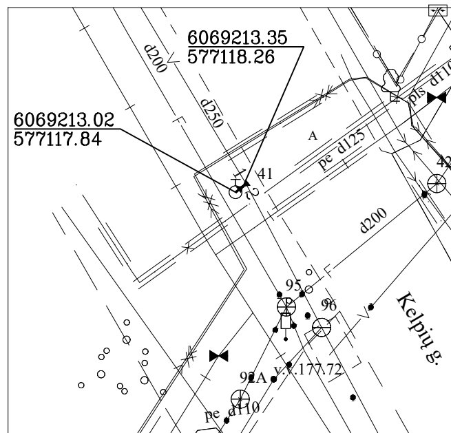
Pririšimo schema
