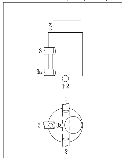
ŠULINIO PJŪVIAI (Matmenys duoti m)
