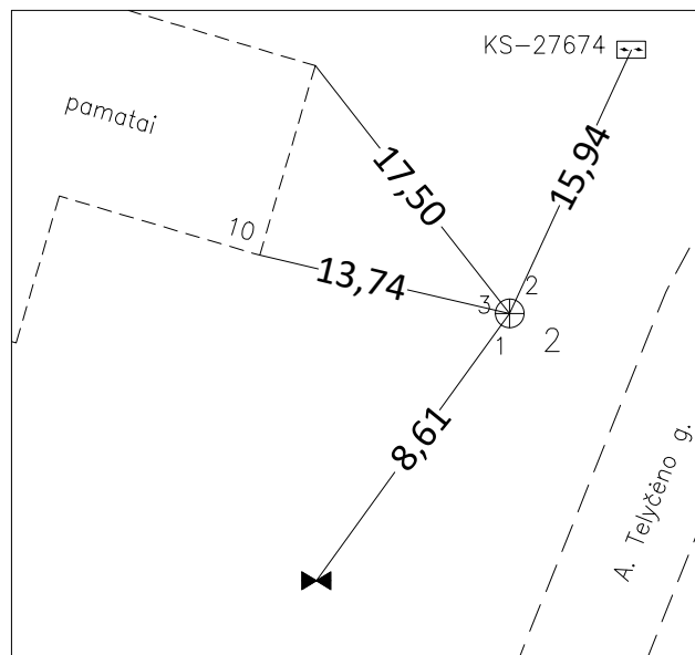
Pririšimo schema
