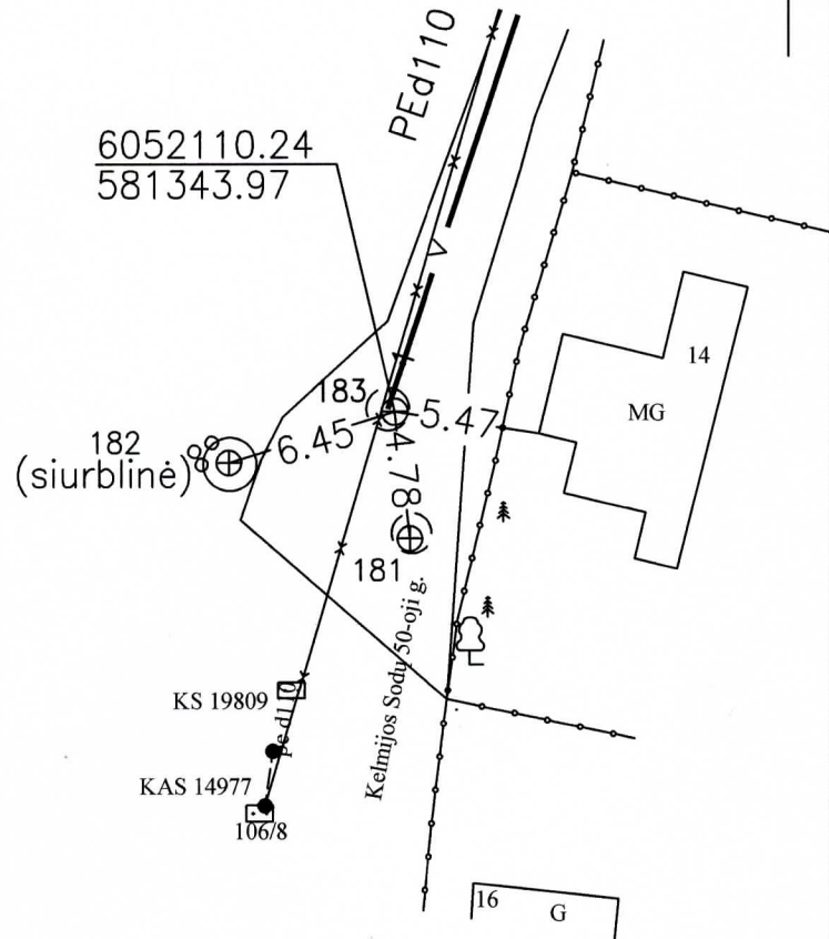
Pririšimo brėžinys
