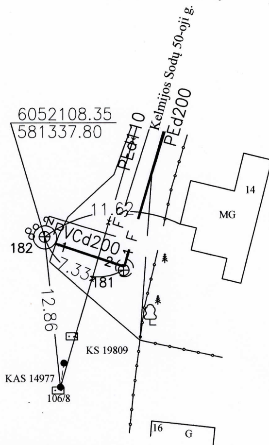
Pririšimo brėžinys
