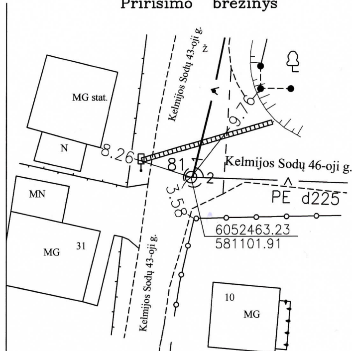
Pririšimo brėžinys
