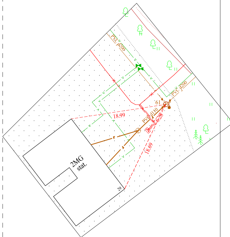
Pririšimo brėžinys
