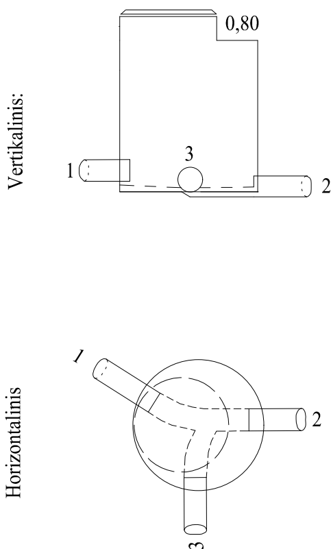
Šulinio pjūviai:
