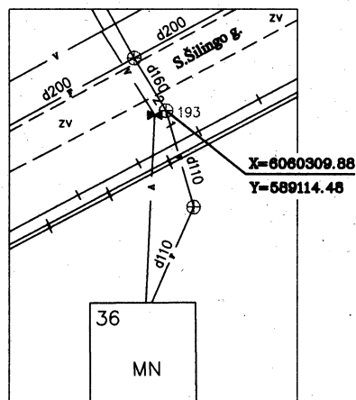
PRIRIŠIMO BRĖŽINYS
