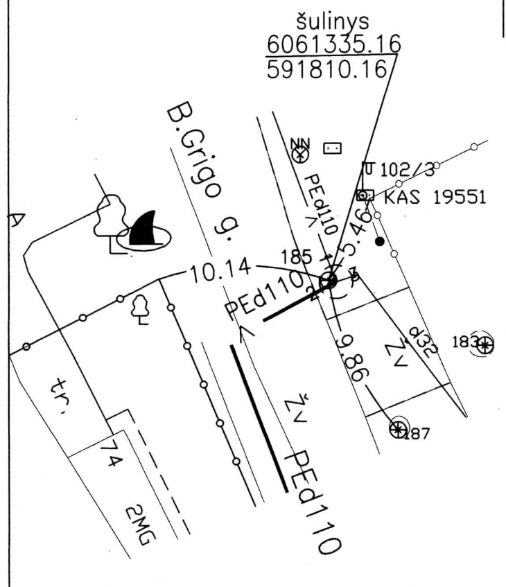
Pririšimo brėžinys
