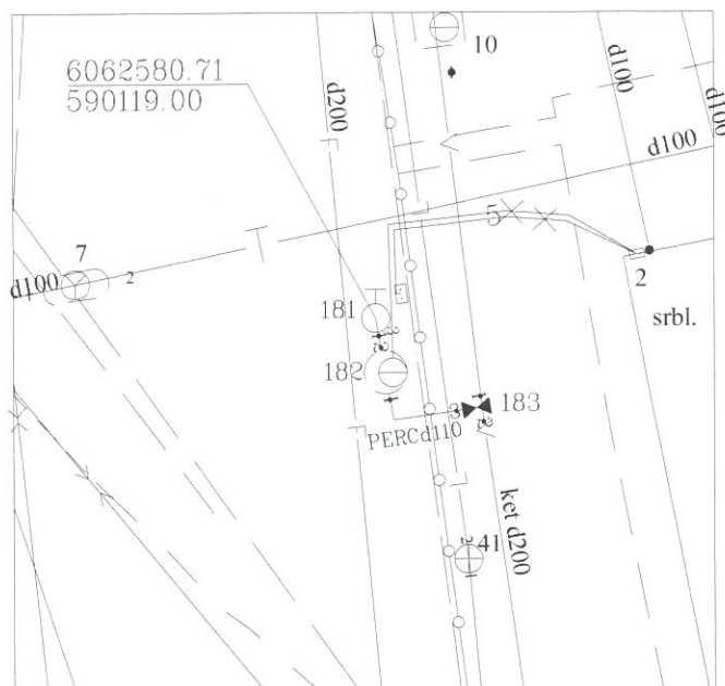
Pririšimo schema
