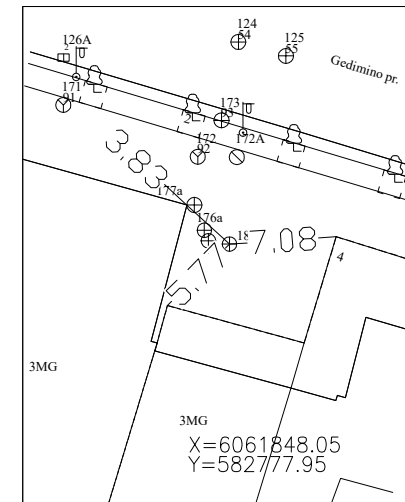
PRIRIŠIMO BRĖŽINYS
