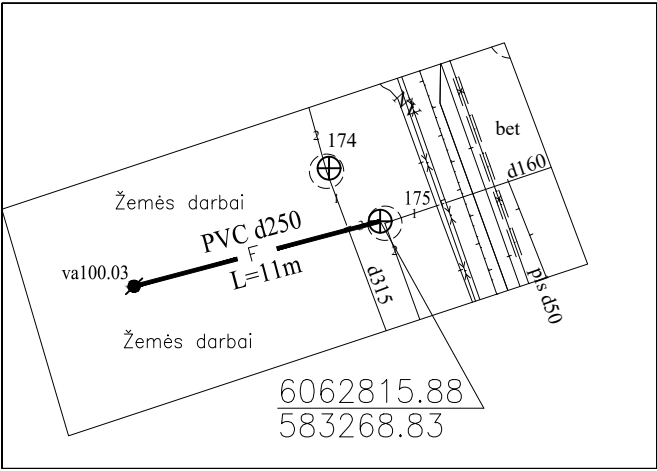
Pririšimo brėžinys
