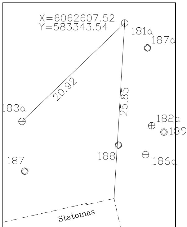
PRIRIŠIMO BRĖŽINYS
