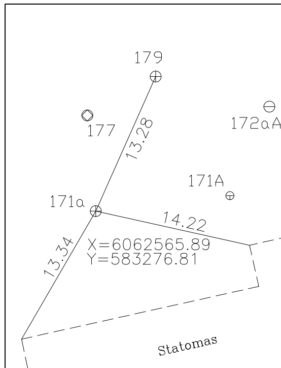
PRIRIŠIMO BRĖŽINYS
