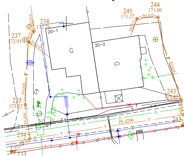
Pririšimo brėžinys
