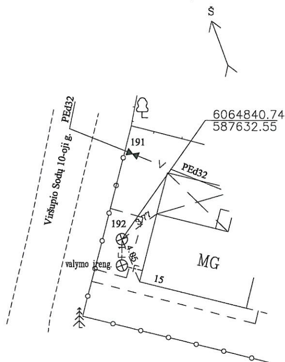
Pririšimo brėžinys
