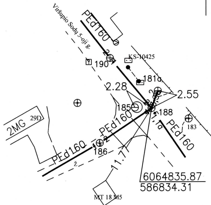
Pririšimo brėžinys
