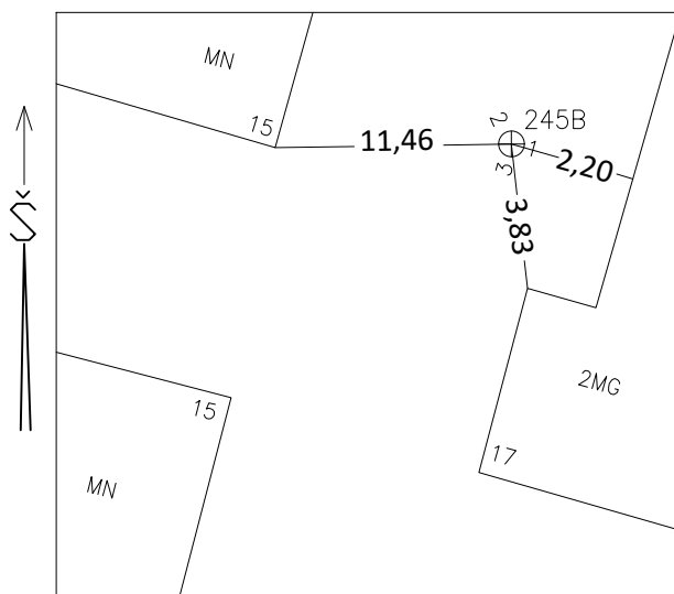
Prišimo schema
