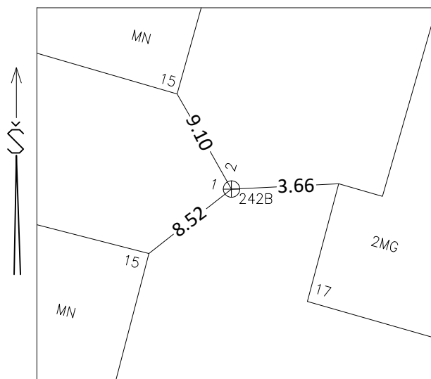
Pririšimo schema
