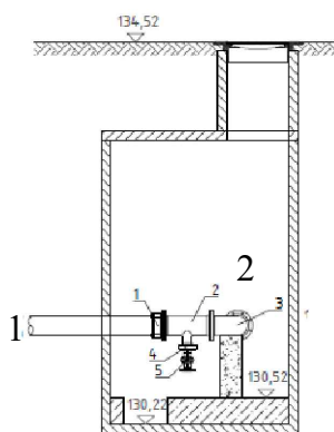
Pjūvis A-A
